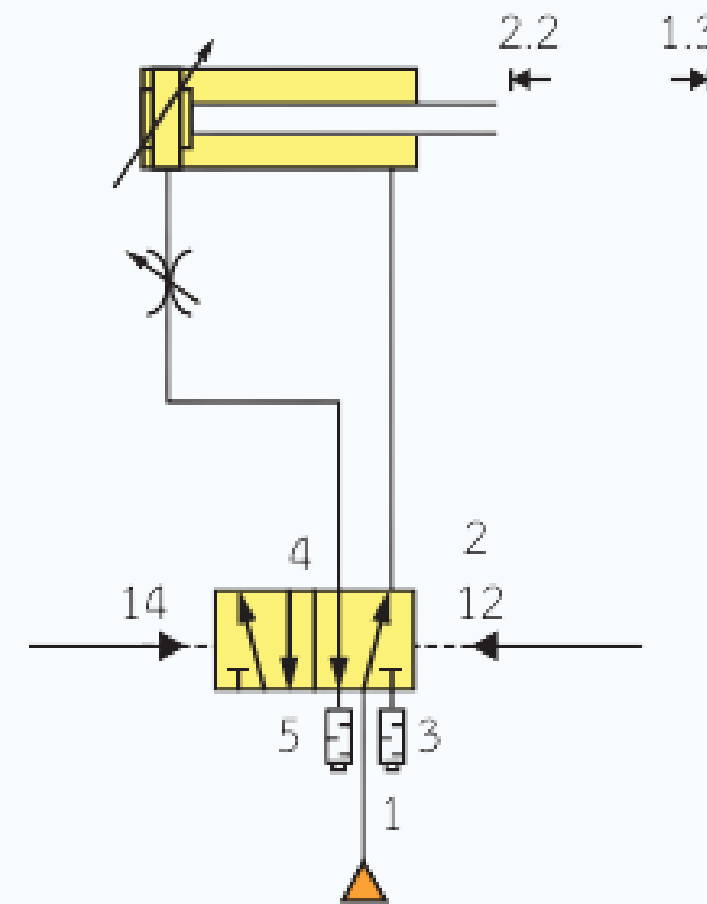
แสดงวงจรนิวเมติกส์ (วงจรกำลัง)
