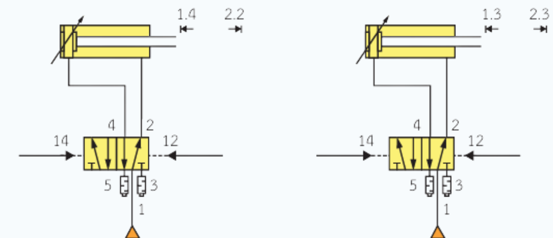
แสดงวงจรนิวเมติกส์ (วงจรกำลัง)
