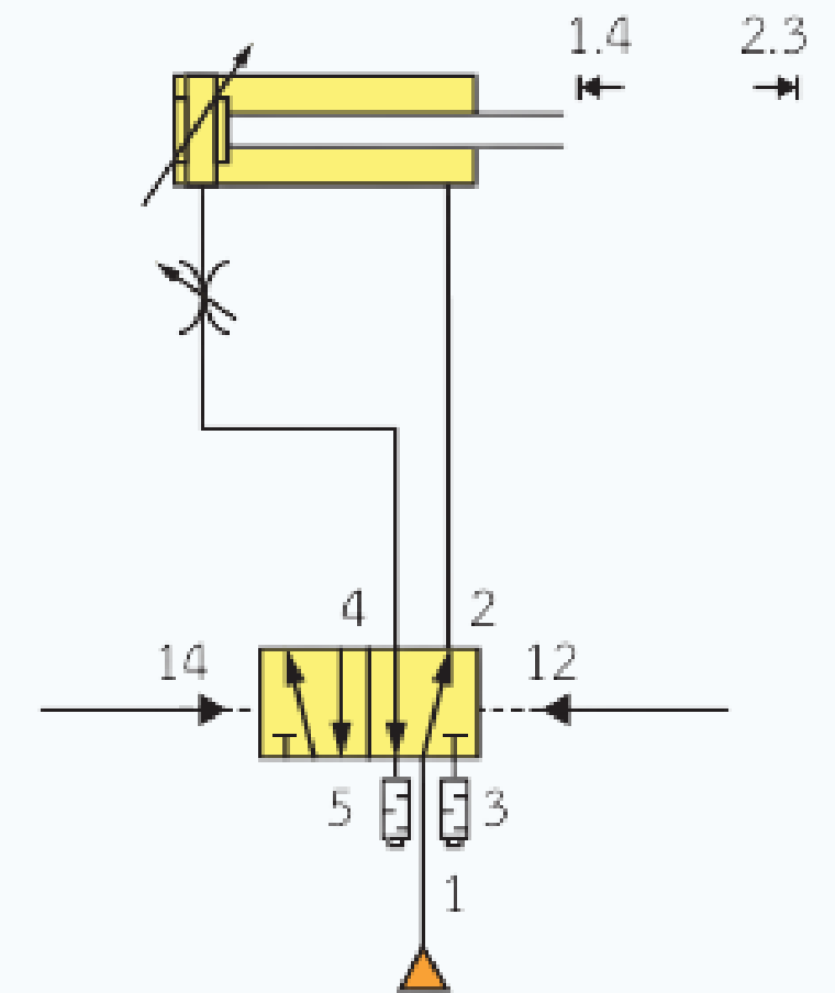
แสดงวงจรนิวเมติกส์ (วงจรกำลัง)
