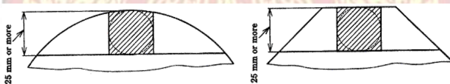
ภาพที่ 10 : ชิ้นงานทดสอบประเภท bar หลังจากทำการกลึงไสแล้ว
