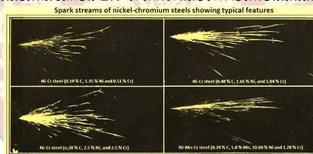
รูปที่ 11 กระแสประกายไฟของเหล็กนิเกิลโครเมียมแสดงลักษณะทั่วไป
