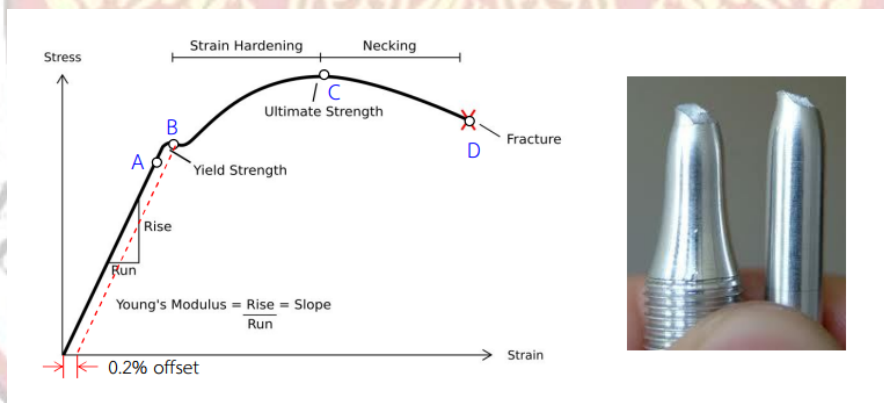
รูปที่ 2 ความสัมพันธ์ระหว่างความเค้น-ความเครียดของวัสดุเหนียวทั่วไป
