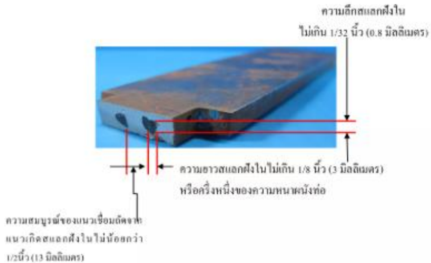
รูปที่ 2.3-10 แสดงขนาดเกณฑ์การยอมรับจุดบกพร่อง ผิวรอยหักขึ้นทดสอบ Nick-break Test
