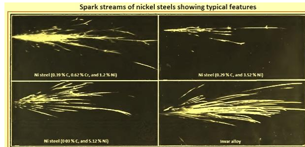
รูปที่ 9 กระแสประกายไฟของเหล็กนิเกิลแสดงลักษณะทั่วไป
