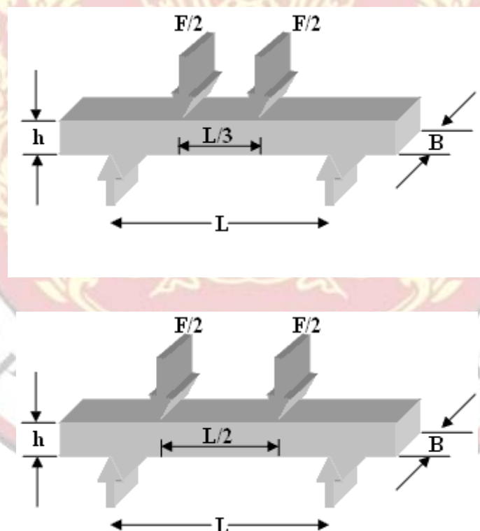
ภาพที่ 3 : การทดสอบการดัดงอแบบ 4 จุด
