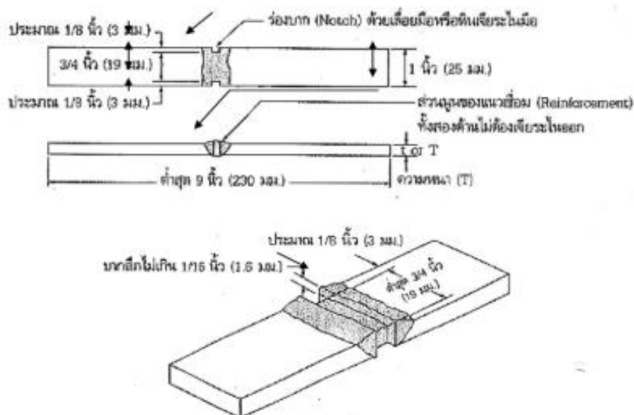
รูปที่ 2.3-3 แสดงชิ้นทดสอบเต็มขนาด (Full-Sized Specimens)
