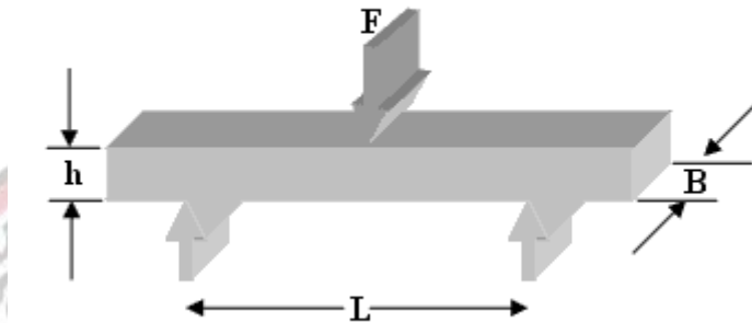
ภาพที่ 2 : การทดสอบการดัดงอแบบ 3 จุด
