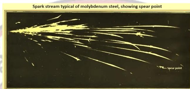
รูปที่ 3 กระแสประกายไฟแบบทั่วไปของเหล็กโมลิบดีนัม
