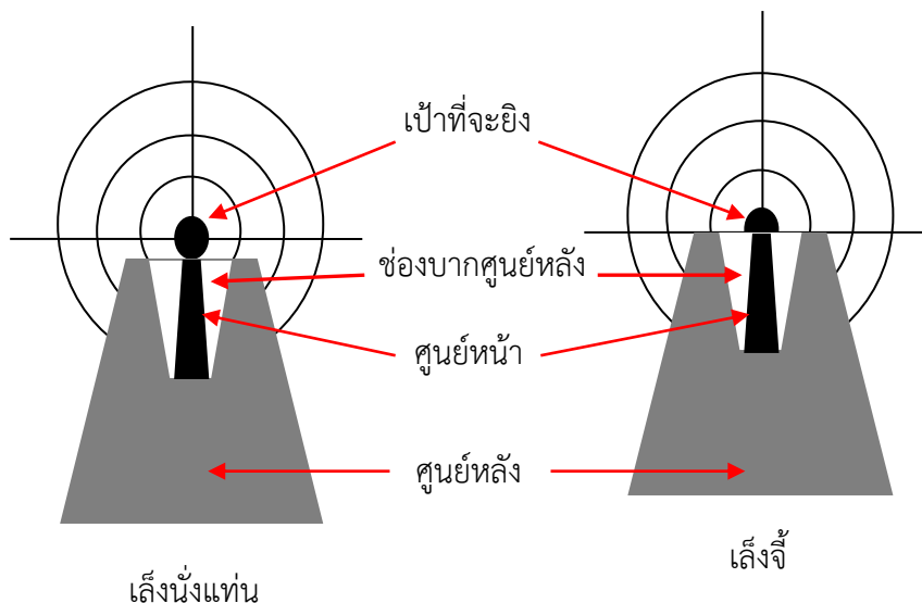
รูปที่ 8 การเล็งเป้าแบบเล็งนั่งแท่นกับแบบเล็งจู้
