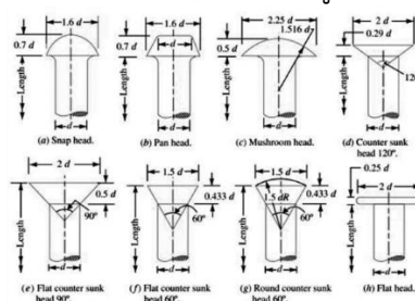
แสดงลักษณะหัวหมุดย้า
