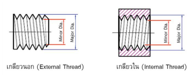
แสดงขนาดเส้นผ่านศูนย์กลางของเกลียว
