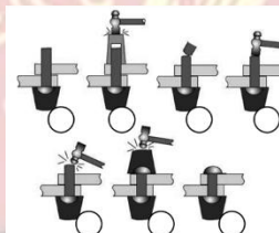
แสดงลักษณะการใช้งานเหล็กย้ำหมุด
