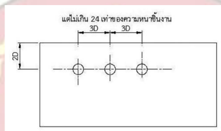
แสดงตำแหน่งเจาะรูชิ้นงานเพื่อย้าหมุด
