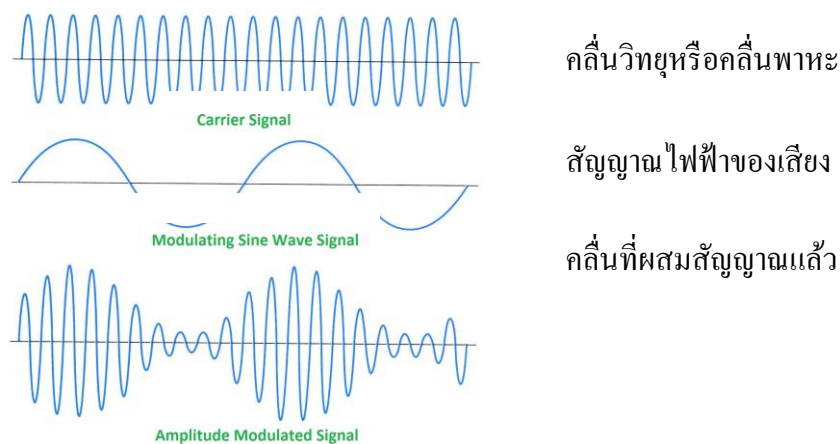
รูปที่ ๘ การผสมสัญญาณระบบ AM
