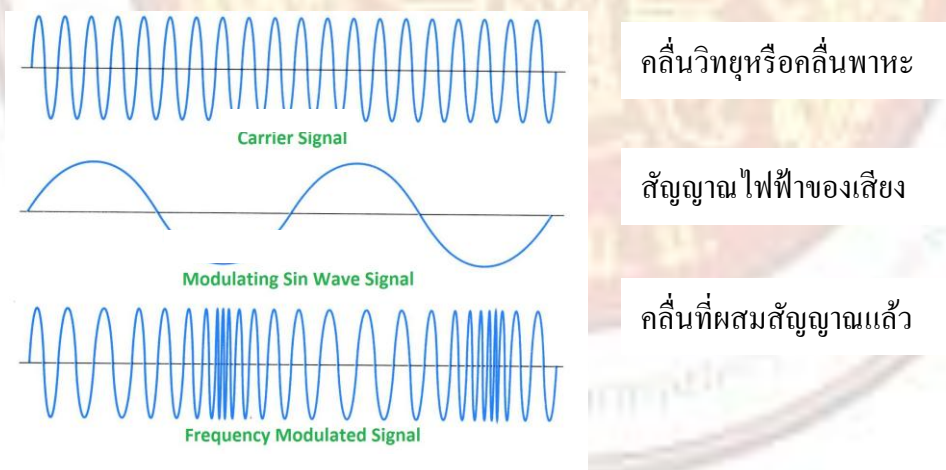
รูปที่ ๙ การผสมสัญญาณระบบ FM
