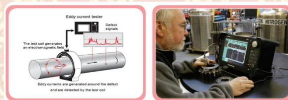
ภาพที่ 11.6 การตรวจสอบด้วยวิธีกระแสไหลวน
