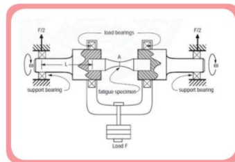
ภาพที่ 11.12 ลักษณะการทดสอบแรงล้า
