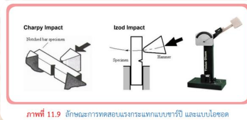
ภาพที่ 11.9 ลักษณะการทดสอบแรงกระแทกแบบชาร์ปี และแบบไอซอด
