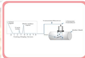
ภาพที่ 11.4 การตรวจสอบด้วยคลื่นอัลตราโซนิก
