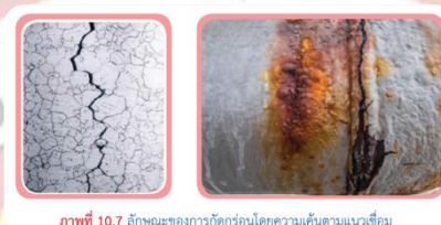
ภาพที่ 10.7 ลักษณะของการกัดกร่อนโดยความเค้นตามแนวเชื่อม
