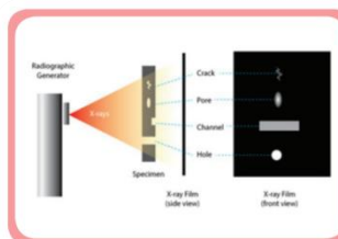
ภาพที่ 11.5 การตรวจสอบด้วยวิธีถ่ายภาพด้วยรังสี
