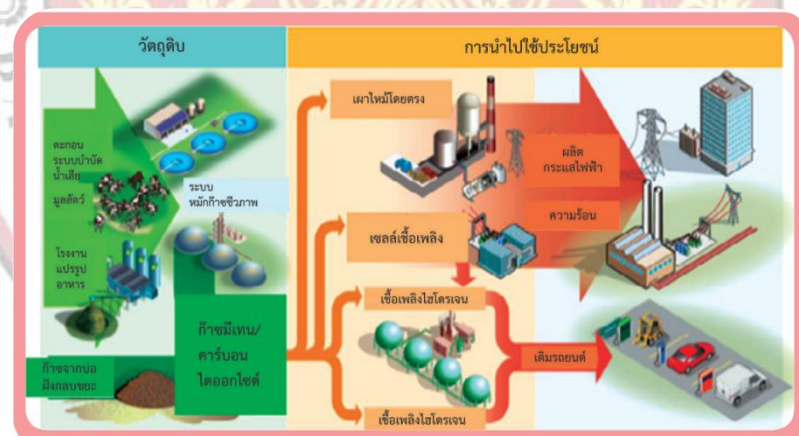
ภาพที่ 6.25 กระบวนการ และการใช้งานแก๊สชีวภาพ
