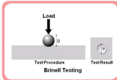
ภาพที่ 11.13 ลักษณะการทดสอบความแข็งแบบบริเนลล์
